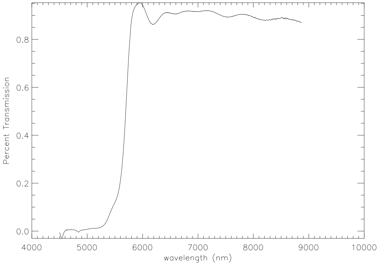
560 Dichroic
